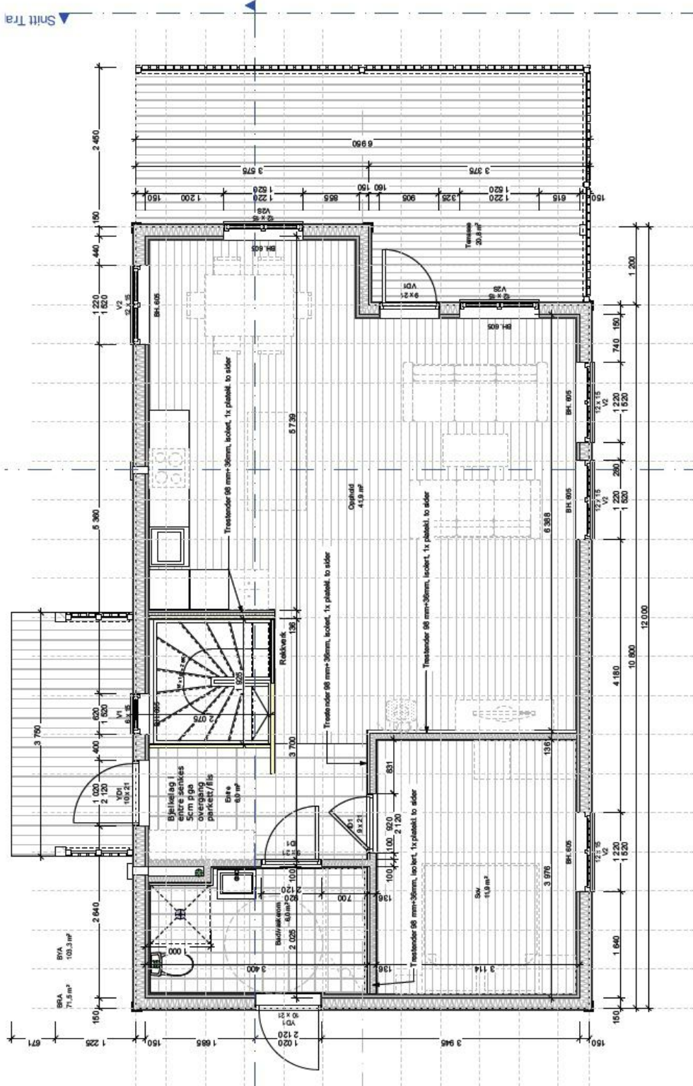
1. Etasje
