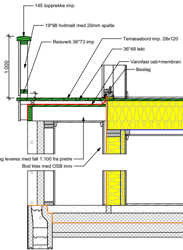
Tett terrasse med bod (Hustype A)
