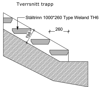
Stigningsforhold tilpasses terrenget.
