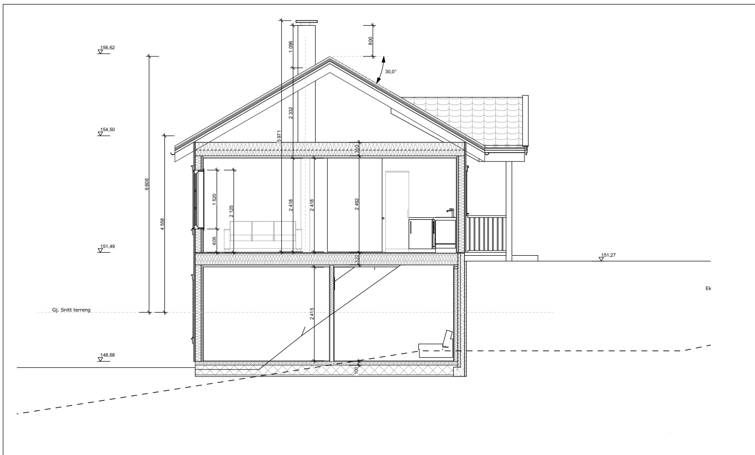
Snitt A
