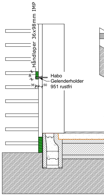
Utvendig trapp inntil vegg
